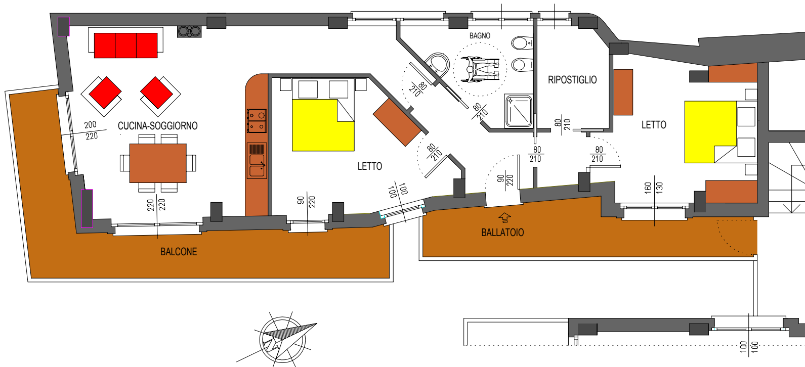
PIANTA PIANO PRIMO TRILOCALE (N.3)
